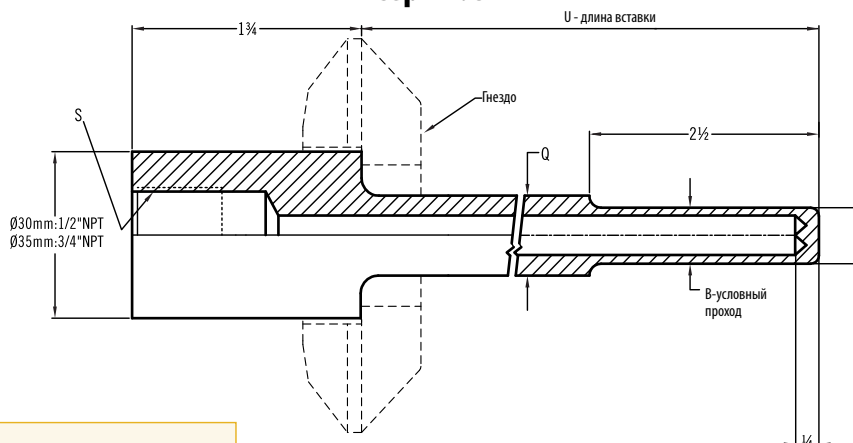
Приварной тип
