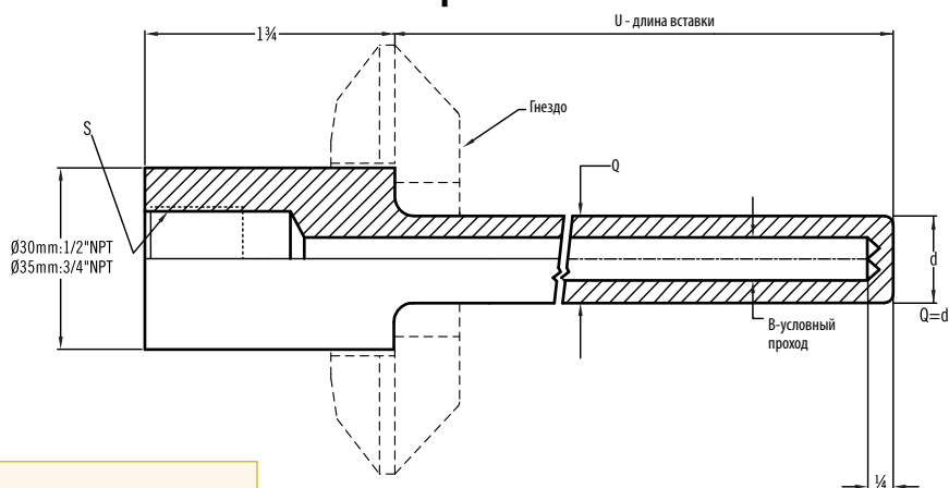
Приварной тип
