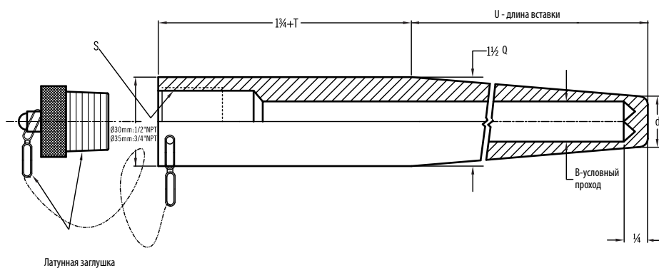
Вварной тип
